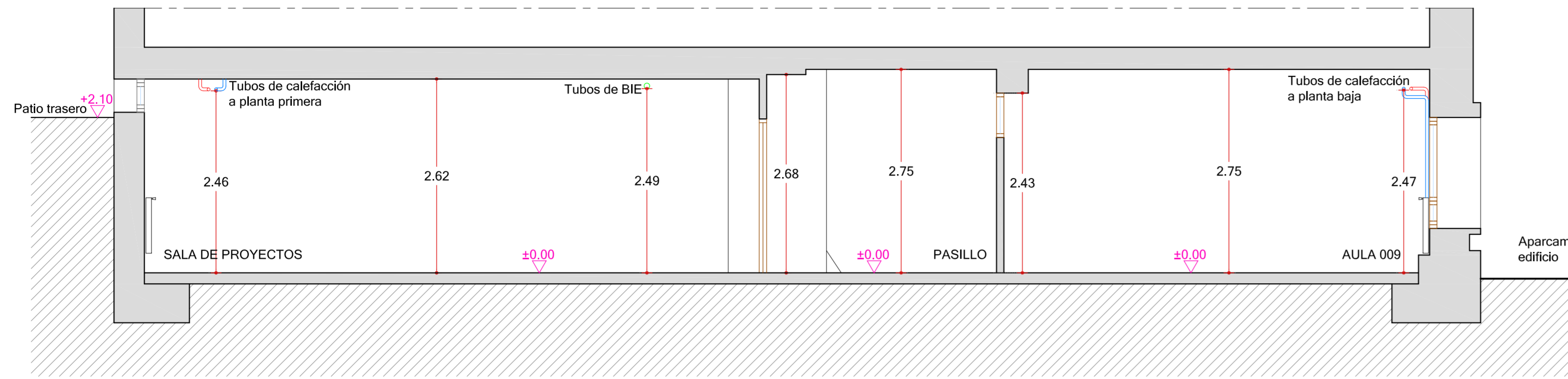
SECCIÓN s1 E: 1/30
